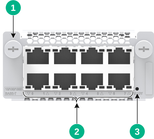
图2-4 NS-HPIM-GT8A-Z 接口模块正视图
