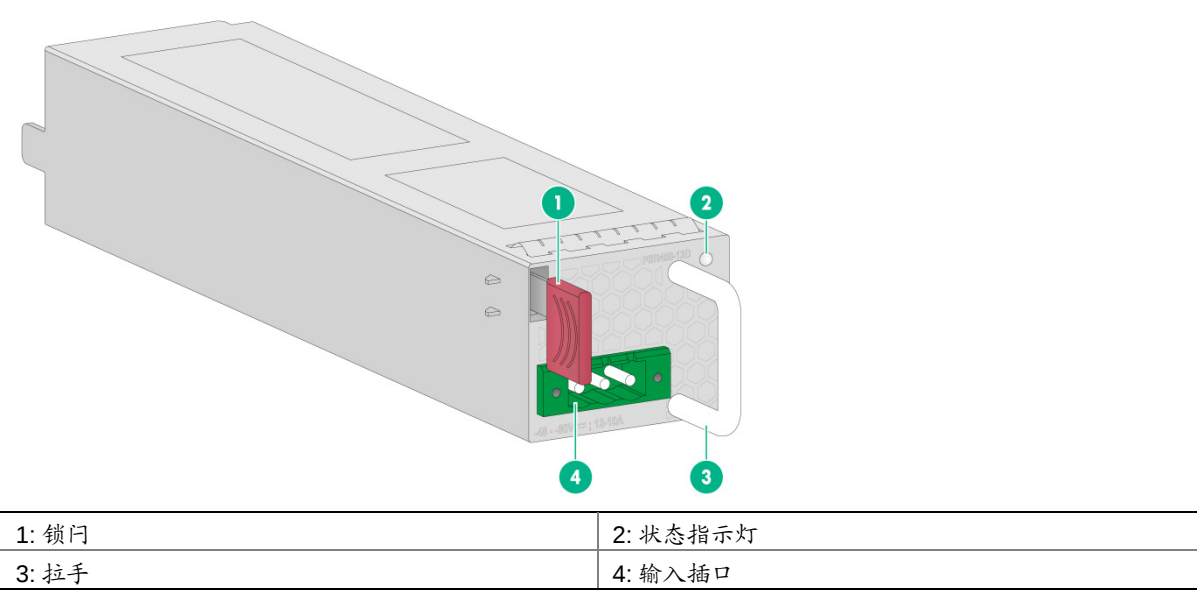
图2-10 直流电源模块正视图
