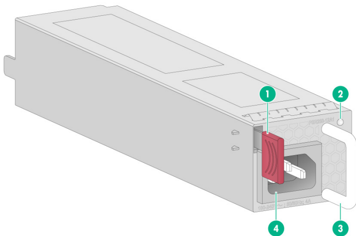
图2-8 交流电源模块正视图
