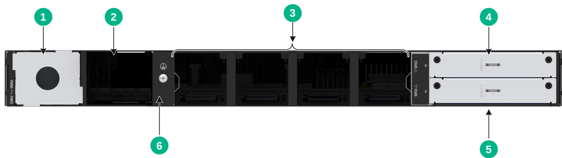
图1-2 设备后视图
