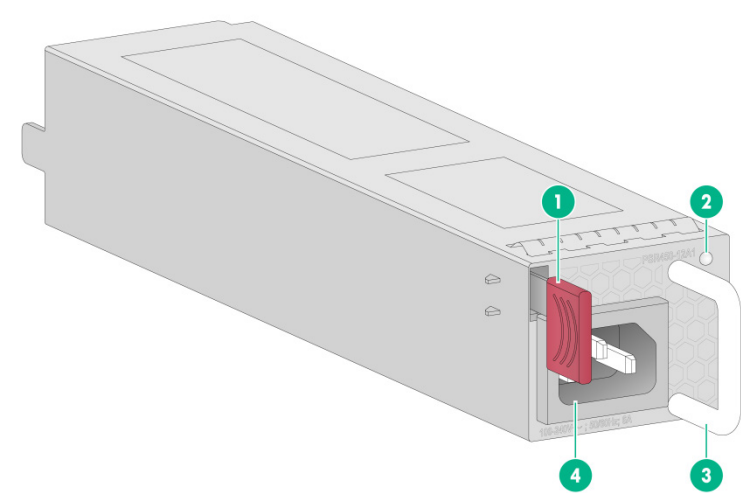
图2-9 交流电源模块正视图
