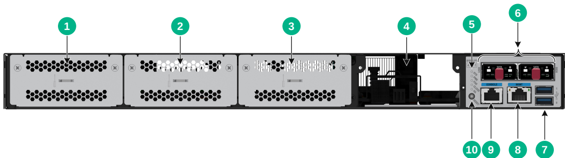
图1-1 设备前视图
